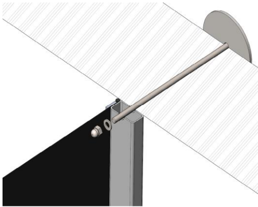
Le mur en béton cellulaire (épaisseur murale 300 mm max.)
