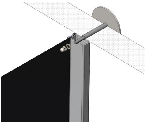
Le mur ISO (épaisseur du mur: 60 mm, 80 mm, 100 mm)
