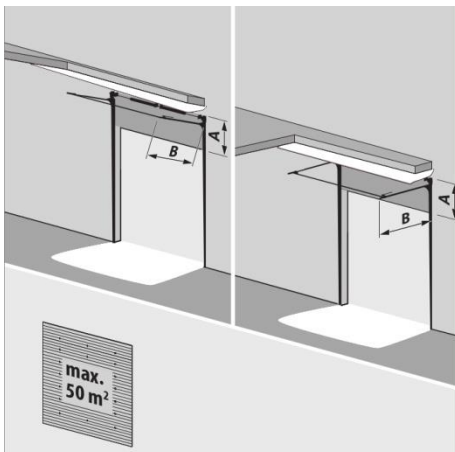
T 240 Système de rails à linteau réduit, câbles glissés à l'intérieur + profilé de support en acier A = 240 mm, B = hauteur du jour + 1000 mm Largeur est max. 7000 mm
