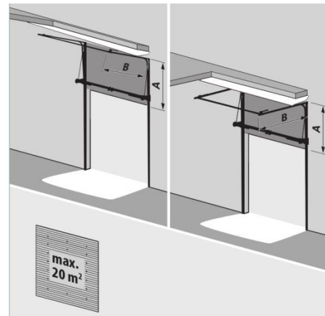
T 400 hF Système de rails levée semiverticale avec axe de ressort surbaissé + profilé de support en acier A = élévation + 200 mm, B = hauteur du jour – élévation + 600 mm Largeur max. 4500 mm, Élévation min. 1450 mm
