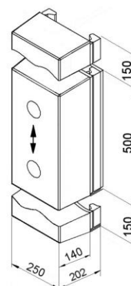
PGB 140 Butoir de quai sur guide verticale (Élément caoutchouc de 140 mm en épaisseur)
