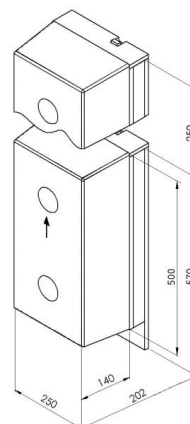
PGV 140 Butoir de quai sur guide verticale (Élément caoutchouc de 140 mm en épaisseur)
