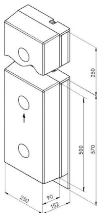
PGV 90 Butoir de quai sur guide verticale (Élément caoutchouc de 90 mm en épaisseur)
