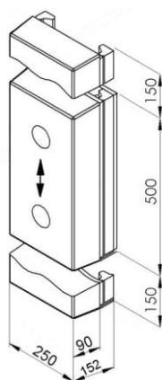
PGB 90 Butoir de quai sur guide verticale (Élément caoutchouc de 90 mm en épaisseur)
