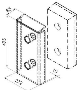
PZPS 90 07 Plaque de protection pour butoir en caoutchouc PGF 90
