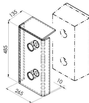
PZPS 140 07 Plaque de protection pour butoir en caoutchouc PGF 140
